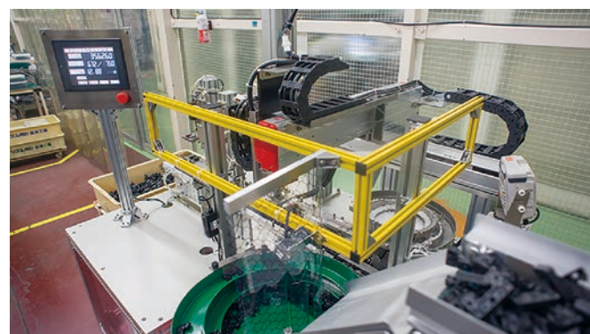
自動検査加工機 Automatic inspection processing machines
